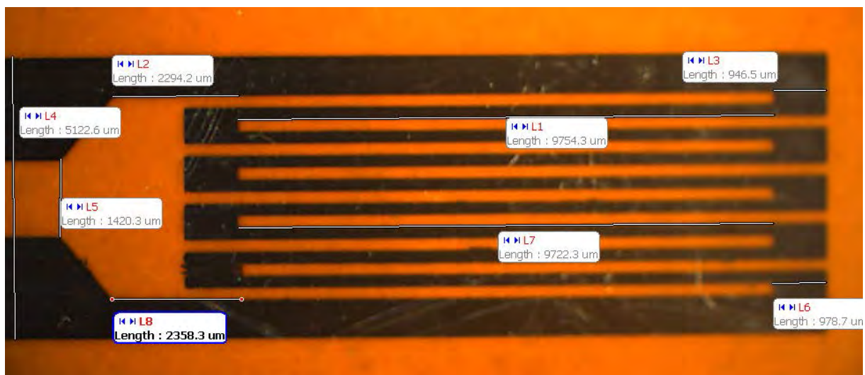
Slika 8. Ostvarene dimenzije odštampanog i sinterovanog senzora,
