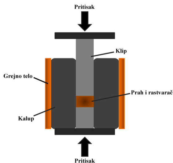
Slika 9. Izgled uređaja za hladno sinterovanje. Preuzeto iz [131].
