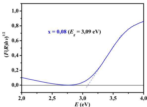
Slika 51. Tauc dijagram za BSSO8-HS-900 sprášeni uzorak.
