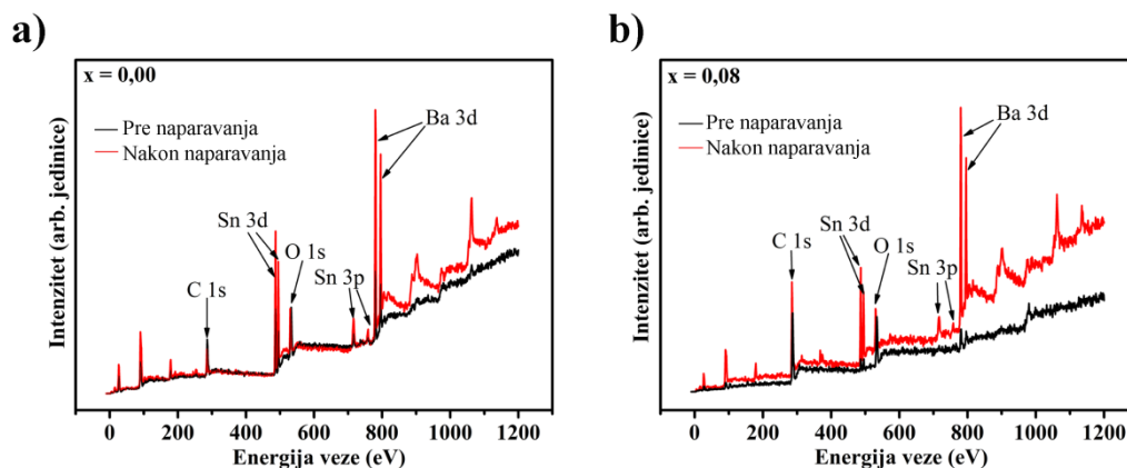
Slika 42. Pregledni XPS spektri za uzorke BSSO x -SPS-1200 za opseg energija veze od 0 do 1200 eV, pre i nakon čišćenja površine uzorka naparavanjem jonima argona: a) x = 0 ; i b) x = 8 .
