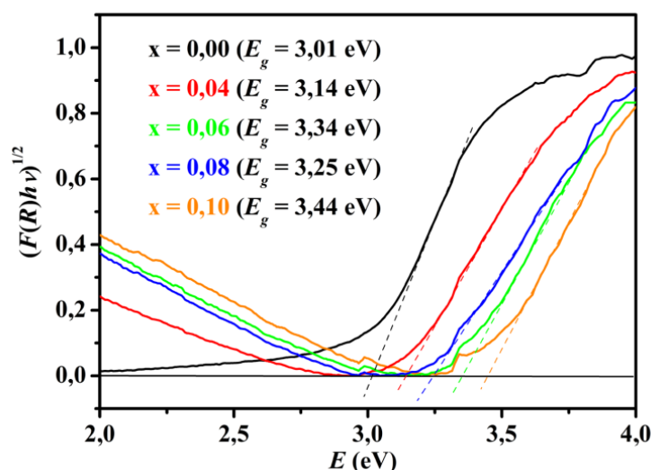
Slika 26. Tauc dijagrami za BSSO x -SPS-1100 ( x = 0, 4, 6, 8, 10 ) sprrašene uzorke.
