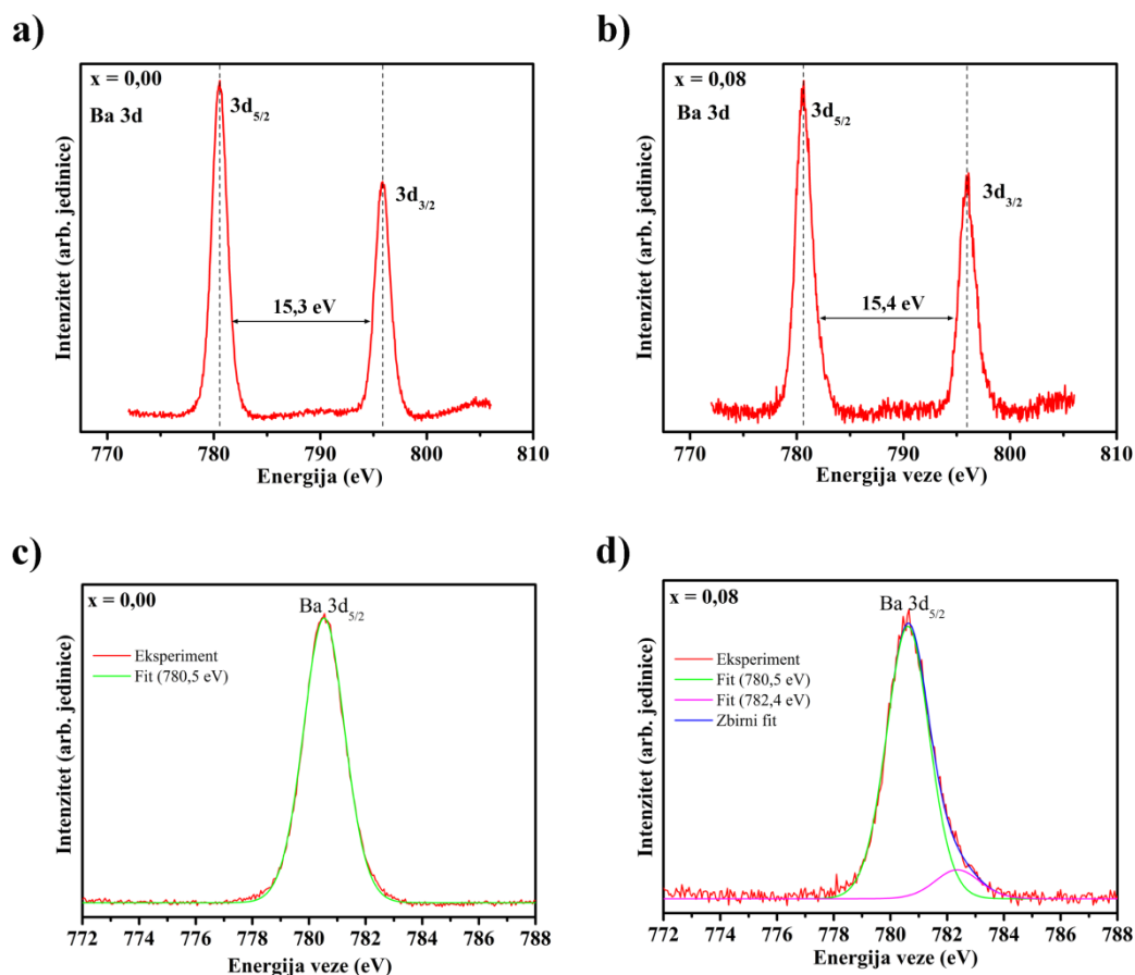
Slika 43. XPS spektri visoke rezolucije za liniju Ba 3d kod uzoraka BSSO x -SPS-1200: a) x = 0 i b) x = 8 . Fitovani XPS spektri visoke rezolucije za liniju Ba 3d 5/2 kod uzoraka BSSO x -SPS-1200: c) x = 0 i d) x = 8 .
