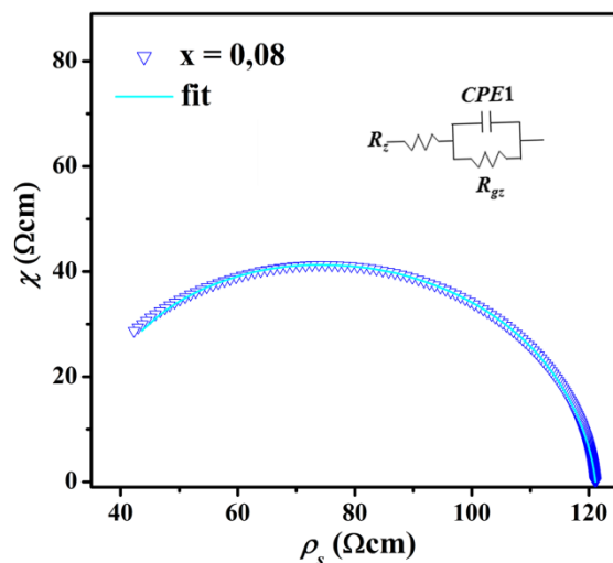
Slika 53. Impedansni spektrar za BSSO8-HS-900 uzorak sa odgovarajućim ekvivalentnim kolom.
