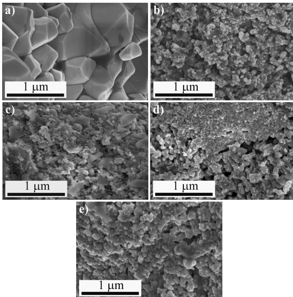
Slika 25. FE-SEM mikrografije urađene na prelomu uzoraka BSSO x -SPS-1100: a) x = 0 ; b) x = 4 ; c) x = 6 ; d) x = 8 ; i e) x = 10 .
