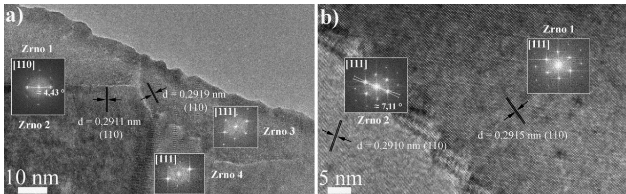
Slika 35. HRTEM mikrografije za BSSO8-SPS-1200 uzorak sa umetnutim FFT za zrna posmatrana iz kristalograskih pravaca: a) [110] i [111]; i b) [111]. Na prikazanim zrnima su izračunata međuravanska rastojanja ( d ) sa odgovarajućih kristalografskih ravni.
