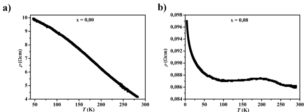
Slika 41. Temperaturna zavisnost električne otpornosti za BSSO _x -SPS-1200 uzorke ispitivana u temperaturnom opsegu: a) od 290 do 50 K za x = 0 ; i b) od 290 do 4 K za x = 8 uzorak.
