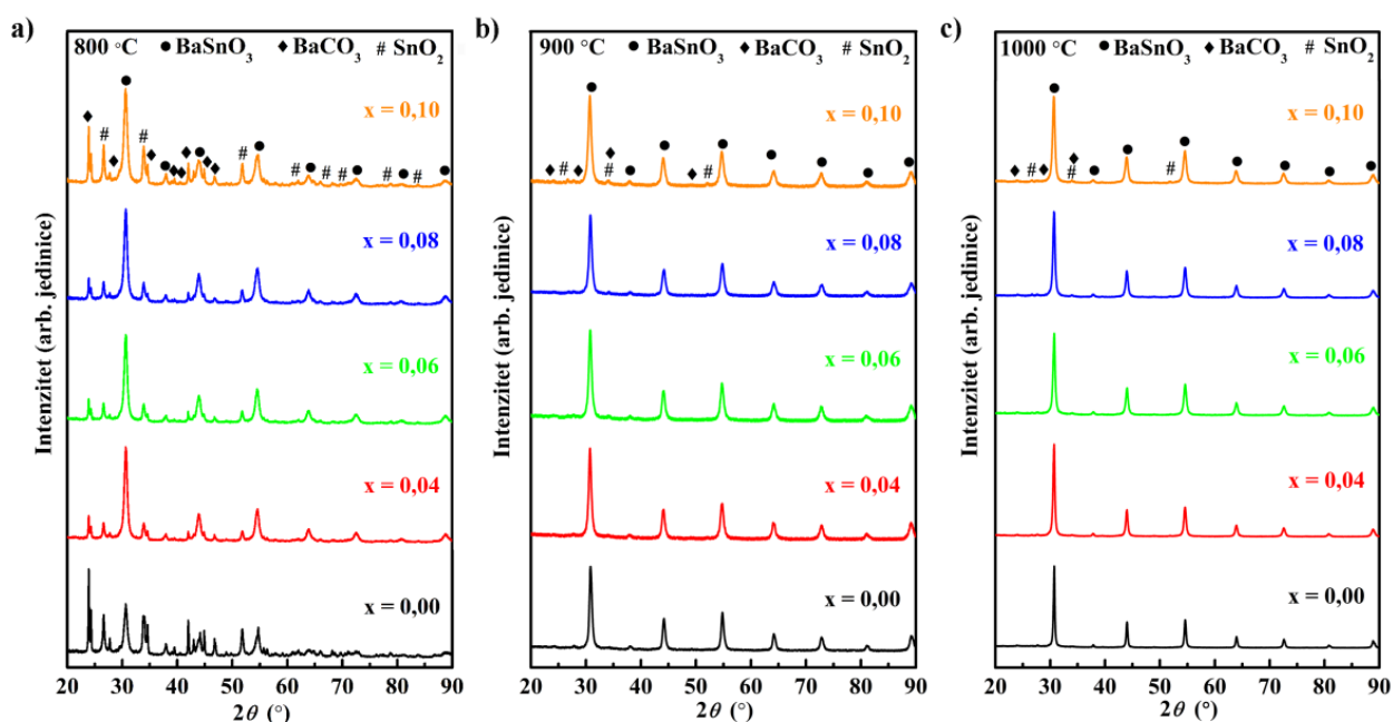
Slika 13. Difraktogrami \text{BSSO}_x ( x = 0, 4, 6, 8 i 10 ) prahova kalciniranih tokom 4 h u atmosferi vazduha na: a) 800 °C; b) 900 °C; i c) 1000 °C.
