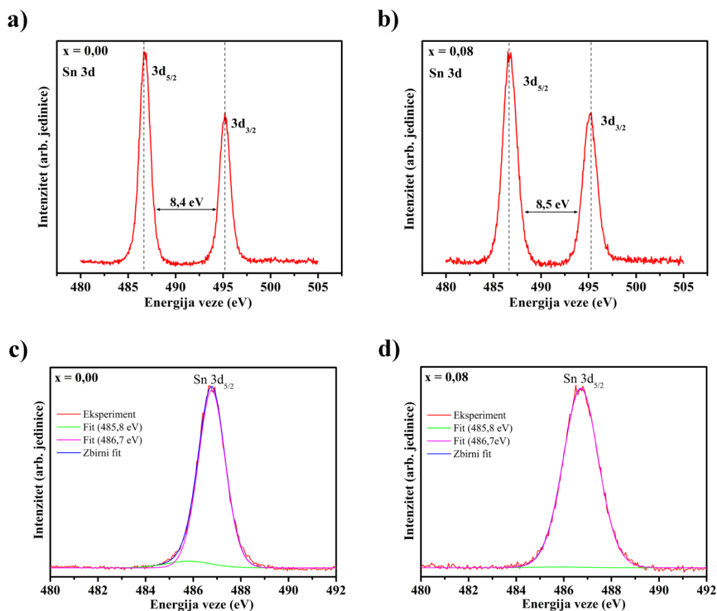
Slika 44. XPS spektri visoke rezolucije za liniju Sn 3d kod uzoraka BSSO x -SPS-1200: a) x = 0 i b) x = 8 . Fitovani XPS spektri visoke rezolucije za liniju Sn 3d 5/2 kod uzoraka BSSO x -SPS-1200: c) x = 0 i d) x = 8 .
