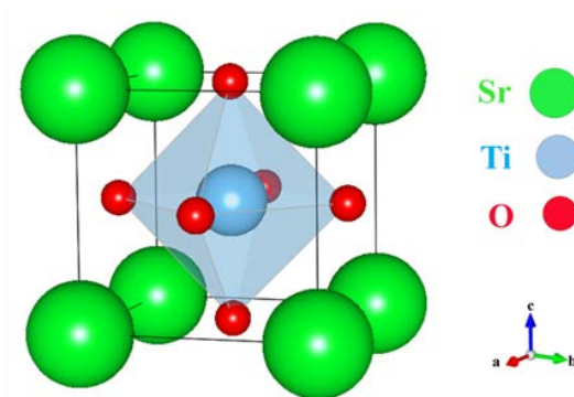
Slika 2. Jedinična ćelija stroncijum-titanata ( SrTiO_3 ) idealne perovskitne strukture
