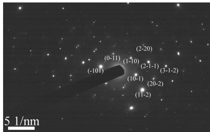
Slika 36. SAED snimak urađen na BSSO8-SPS-1200 uzorku.
