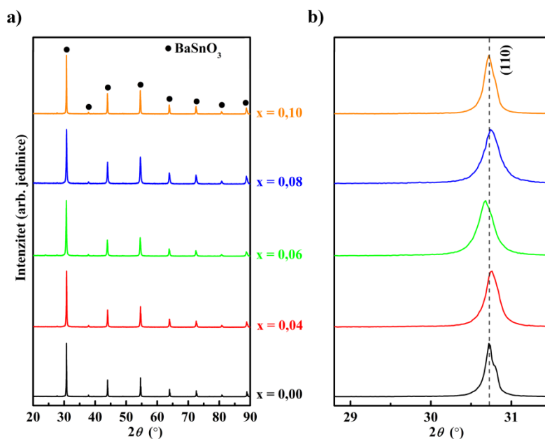
Slika 24. a) Difraktogrami BSSO x -SPS-1100 ( x = 0, 4, 6, 8, i 10 ) sprášenih uzoraka.
