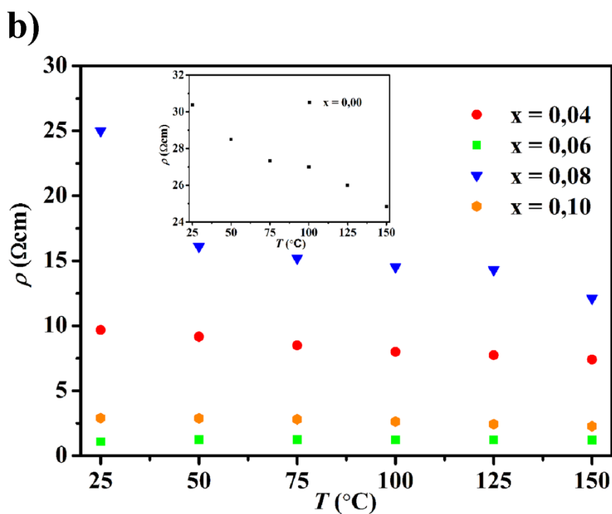
Slika 22. a) I - U karakteristika za BSSO x -KS-1600 [ x = 0 (umetnut grafik); x = 4, 6, 8 i 10 ] keramičke uzorke na sobnoj temperaturi. b) Temperaturna zavisnost specifične otpornosti za iste uzorke u opsegu od 25 do 150 ^{\circ}\text{C}
