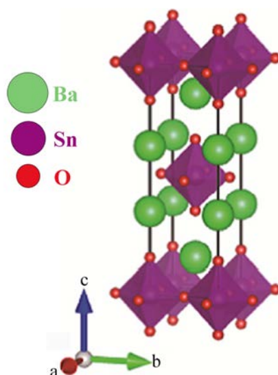
Slika 30. Kristalna struktura barijum-ortostanata, \text{Ba}_2\text{SnO}_4 . Preuzeto iz [152].
