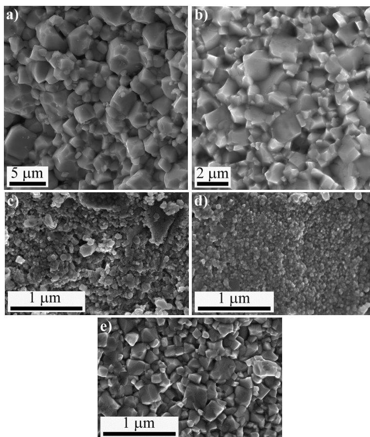
Slika 32. FE-SEM mikrofografije urađene na prelomu uzoraka BSSO x -SPS-1200:
