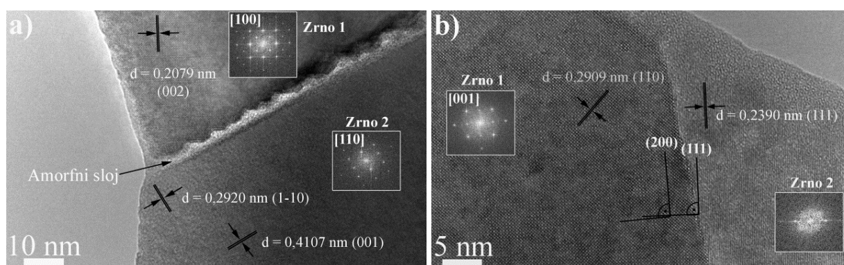
Slika 34. HRTEM mikrografije za BSSO _x -SPS-1200 uzorke sa umetnutim FFT za zrna posmatrana iz kristalografskih pravaca: a) [100] i [110] za x = 0 ; i b) [001] za x = 4 . Na prikazanim zrnima su izračunata međuravanska rastojanja ( d ) sa odgovarajućih kristalografskih ravni. Za x = 0 uzorak prikazan je amorfni sloj u oblasti granice zrna.
