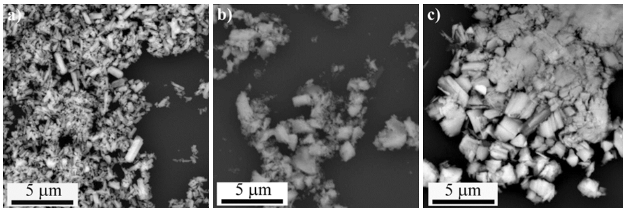
Slika 12. SEM mikrografije polaznih komponenata: a) \text{BaCO}_3 ; b) \text{Sb}_2\text{O}_3 ; i c) \text{SnO}_2 .
